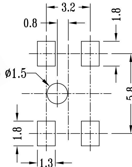
P.C.B LAYOUT
